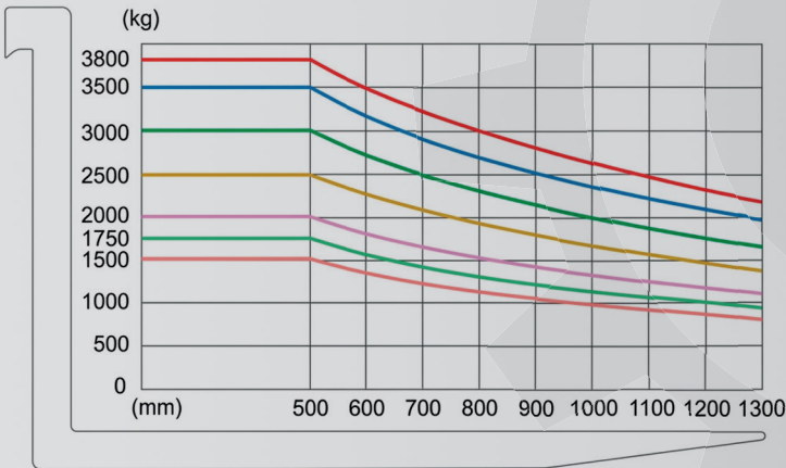
GRÁFICO DE CARGA LINHA FD SERIES
